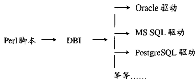
图 13-2 Perl DBI 系统的整体结构图
